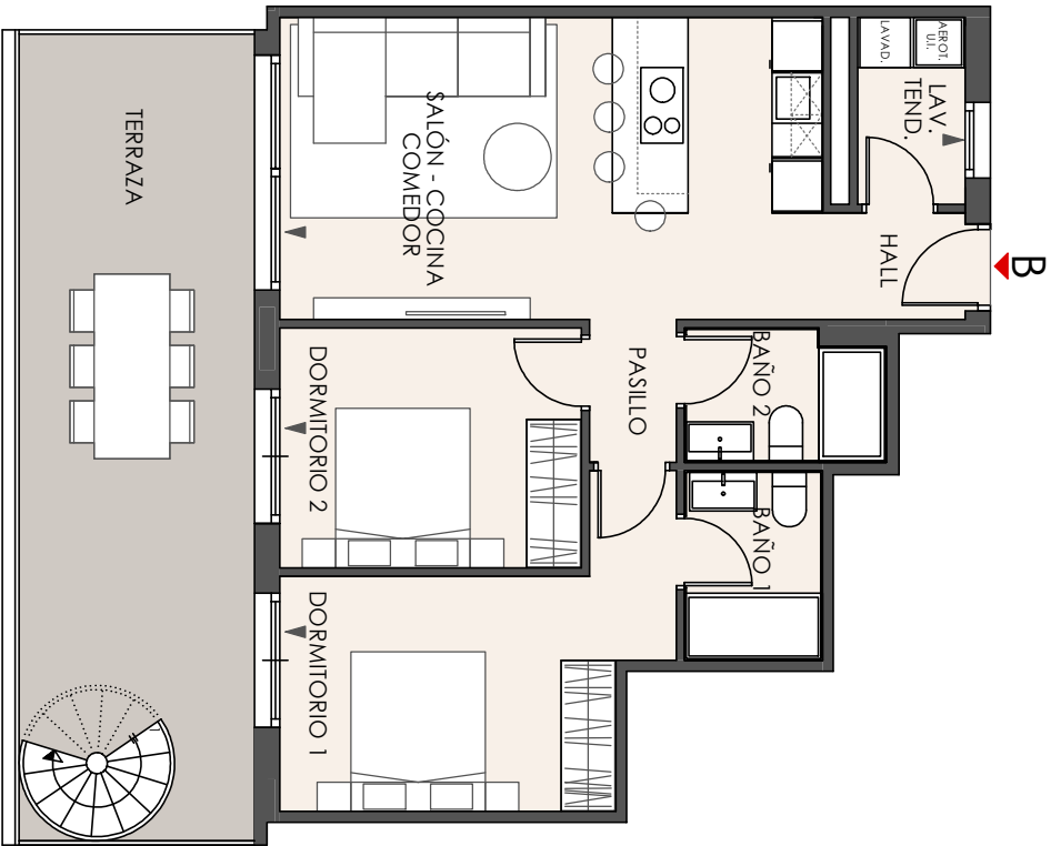
PLANTA 3º
