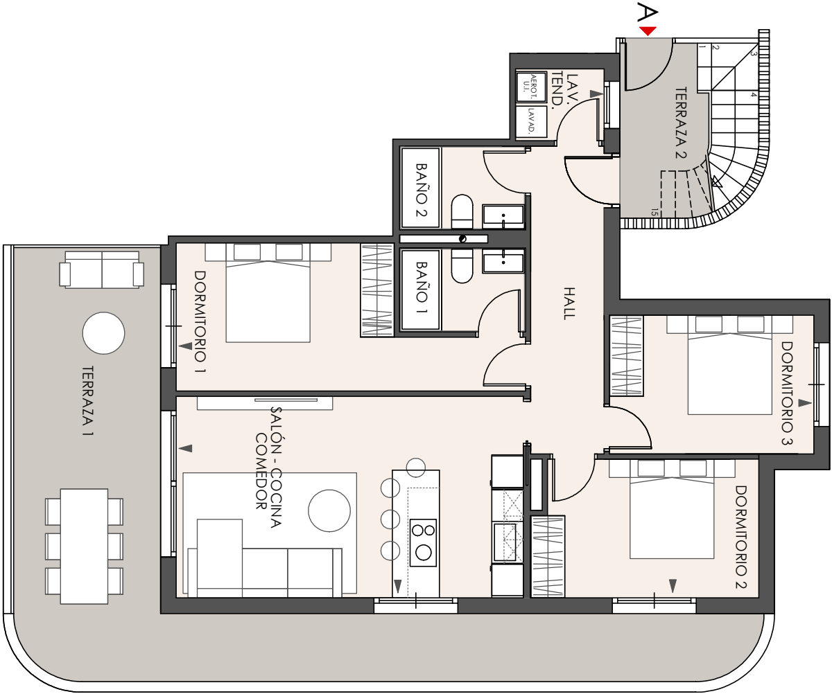
PLANTA 3º
